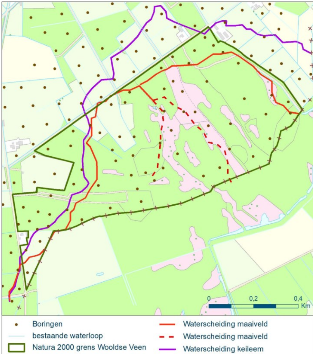
Figuur 3.5. Ligging waterscheiding op basis van het keilempakket en van de maaiveldhoogte.
